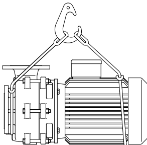
Abb. 2.1a Pumpe und Motor
